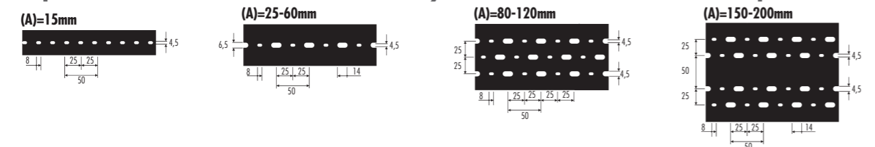
Disposizione fori sul fondo/Sizes and layout of holes on the bottom: Tipo E - E/4
