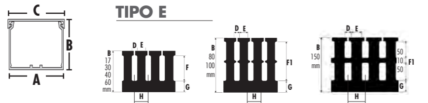
Disposizione fori sul fondo/Sizes and layout of holes on the bottom: Tipo E - E/4
